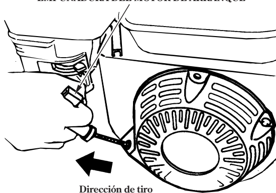
EMPUÑADURA DEL MOTOR DE ARRANQUE
