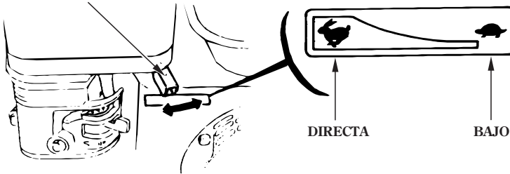
PALANCA DEL ACELERADOR
